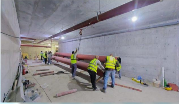
شبكة المياه المبردة وشبكة المياه المركزية جامعة الملك سعود
